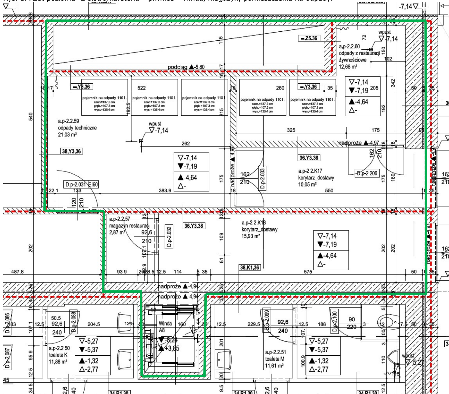
Rys. 1. Rzut poziomu -2 bistro/kafeteria – piwnice – winda, magazyn, pomieszczenia na odpady.
