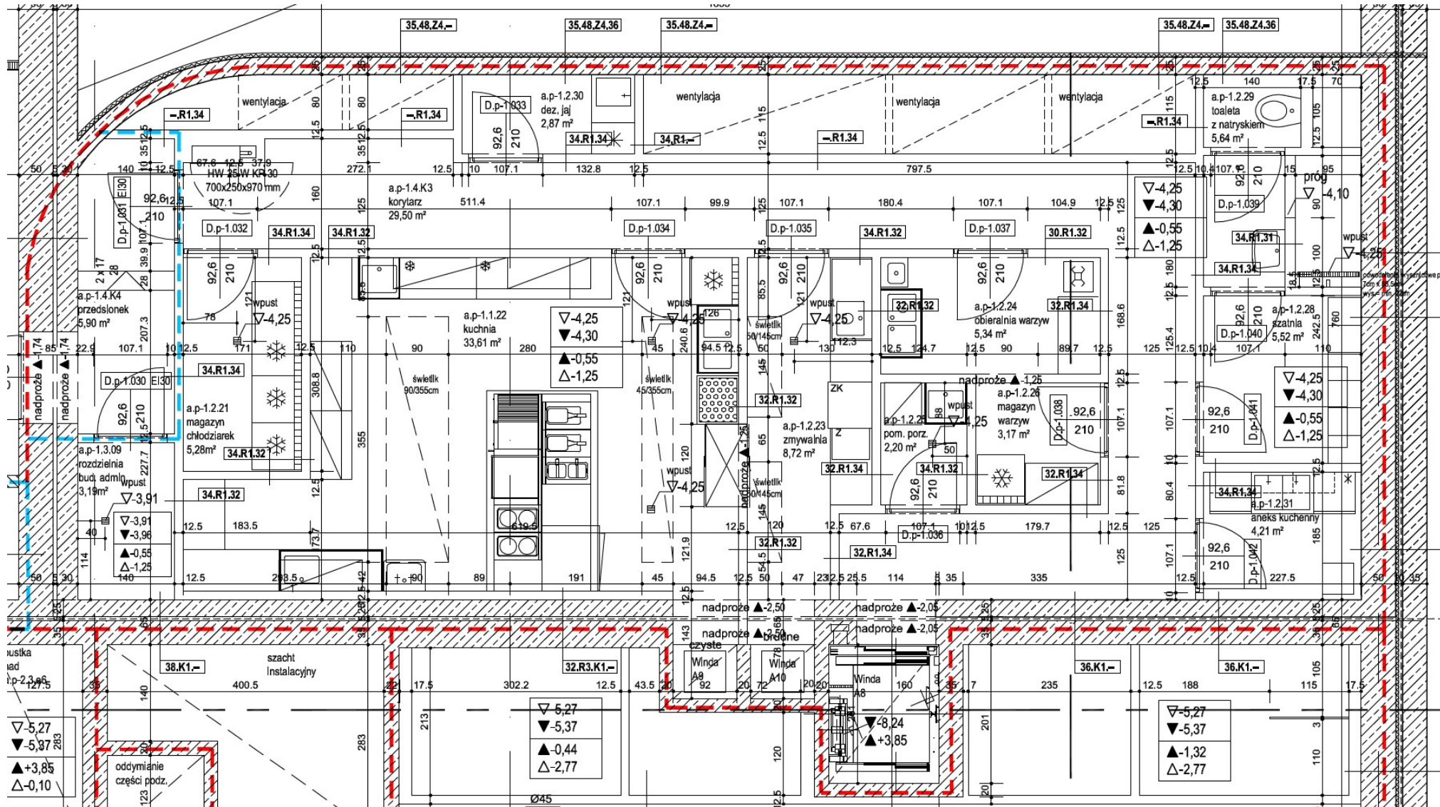
Rys. 2. Rzut poziomu -1 bistro/kafeteria – zaplecze kuchenne.
