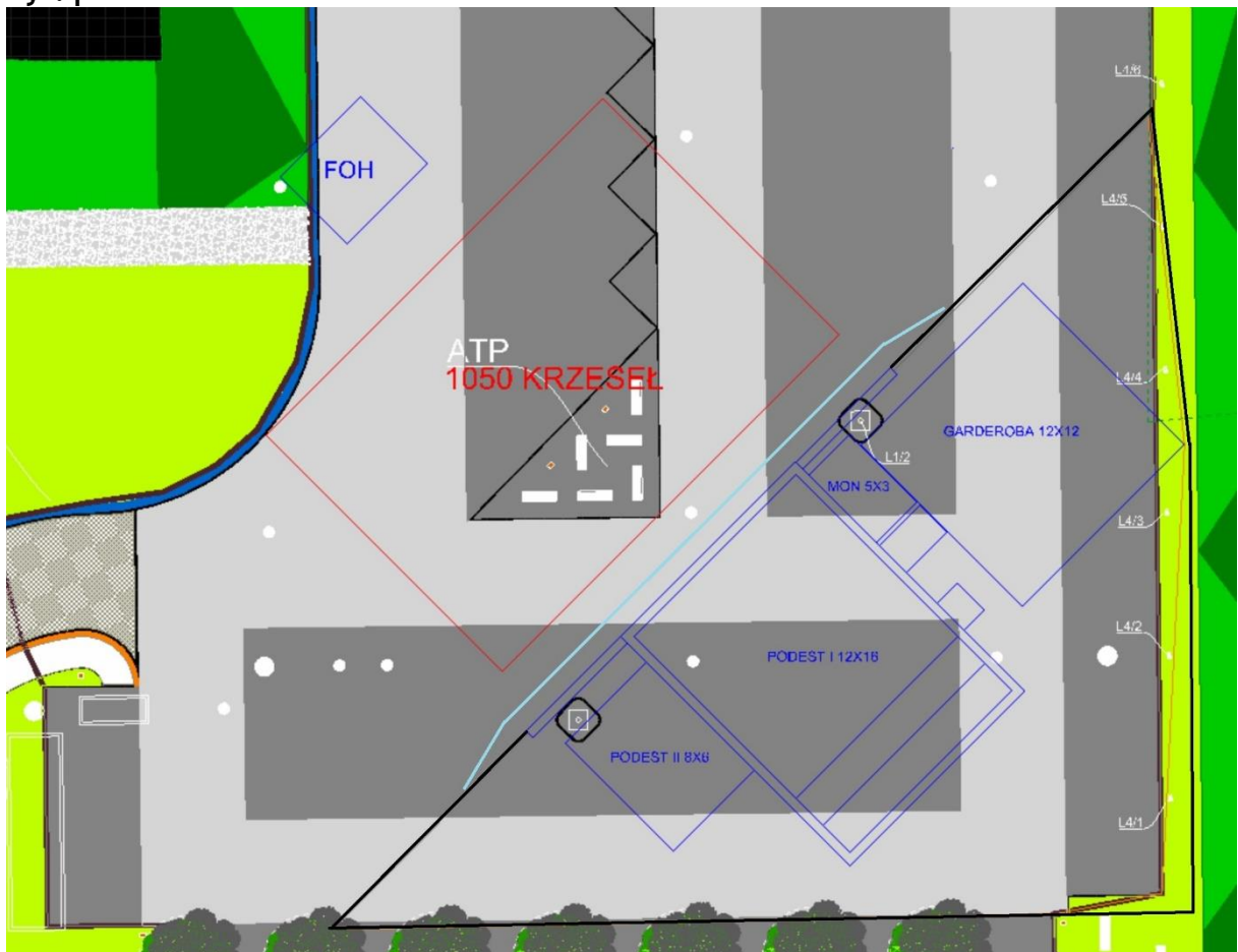
Rys. plan rozmieszczenia techniki
