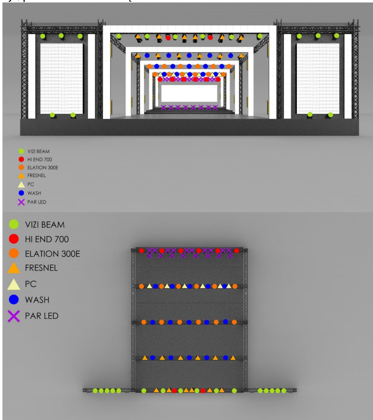
Rys. plan rozmieszczenia urządzeń
